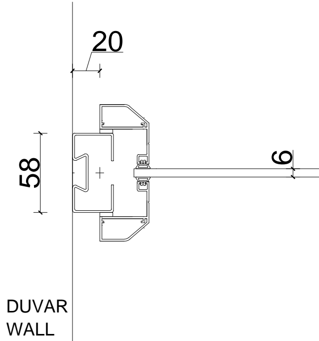
SINGLE GLASS WALL CONNECTION DETAILS TEK CAMLI MODÜL DUVAR BAĞLANTI DETAYI
