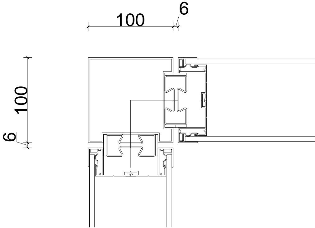
90 CORNER CONNECTION DETAIL KÖŞE BİRLEŞİM BAĞLANTI DETAYI
