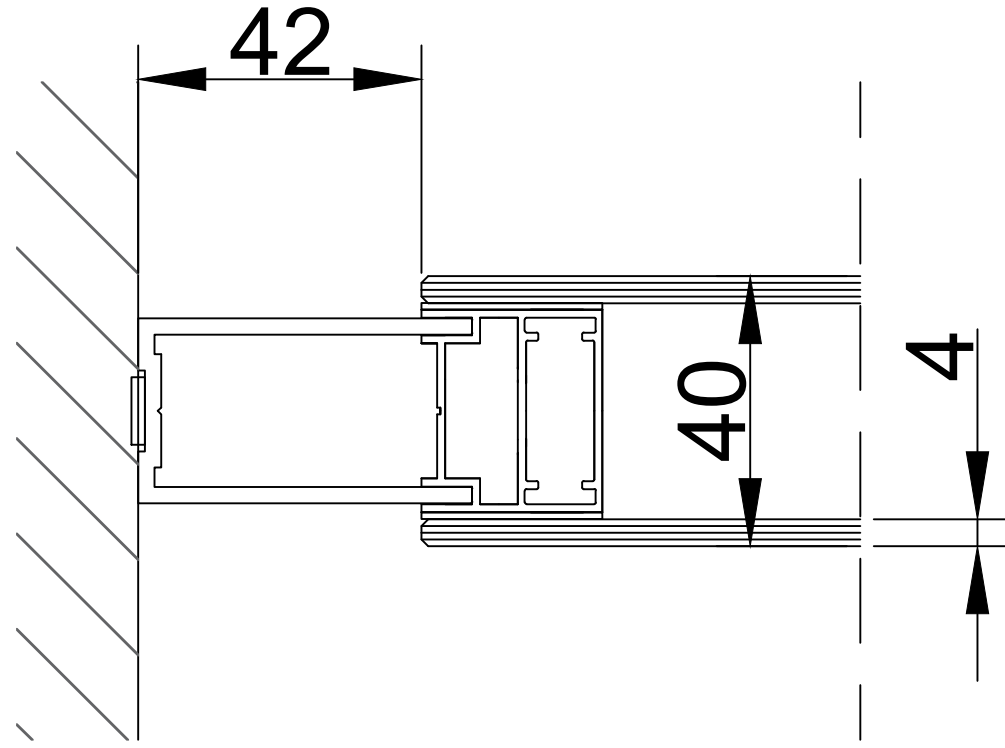
DUVAR BAŞLANGIÇ DETAYI
