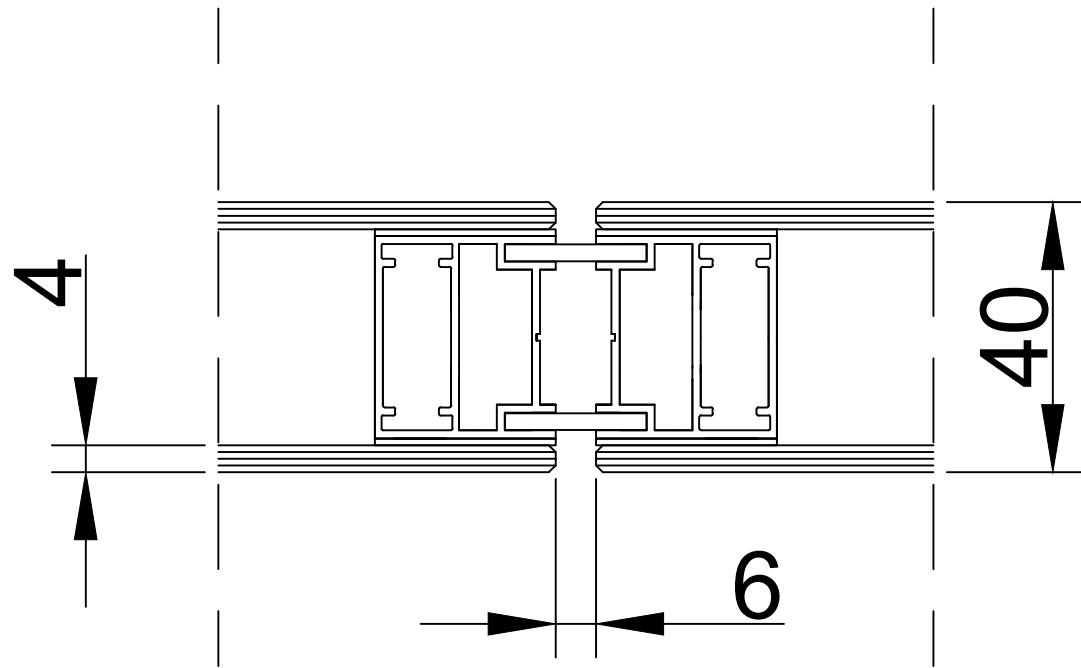
CAM - CAM BİRLEŞİMİ
