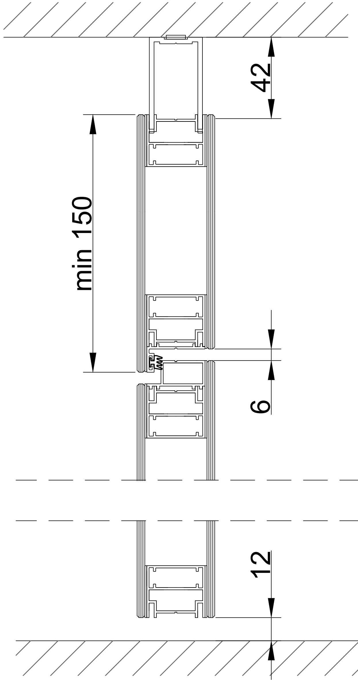
KAPI SİSTEM KESİTİ
